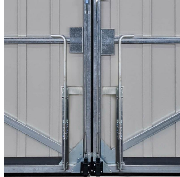
Türstopper (bei Sonderausführung) 500mm
